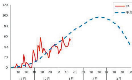
図1 積雪状況推移 (2019~2020新篠津アメダス)
