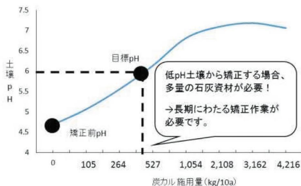
図2 畑地における土壌pHの上昇推移 (実測値により作成した緩衝曲線より)
