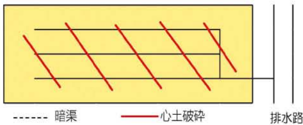
図1 心土破碎の施工例
