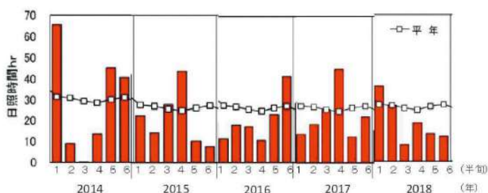
図1 過去5年間の6月の日照時間 (新篠津アメダス)
