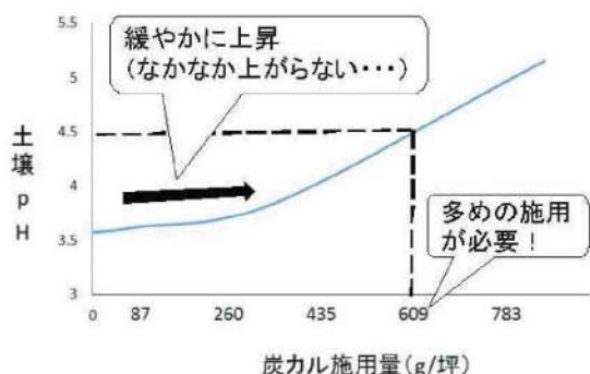
図2 水稲育苗ハウスにおけるpHの上昇推移 (実測値より作成した緩衝曲線より)
