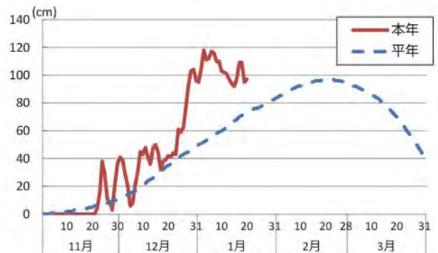
積雪状況推移(2018~2019年新篠津アメダス)
